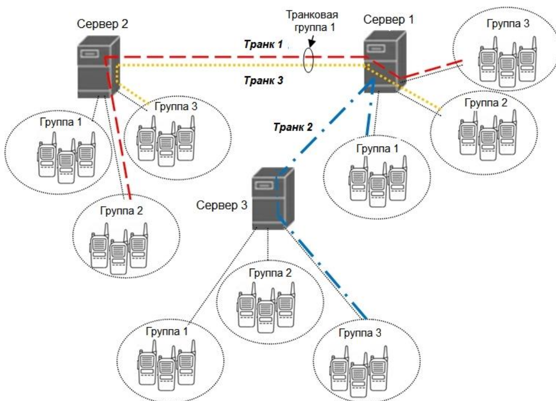
Рис. 2: Мультисерверная система с общими абонентскими группами
