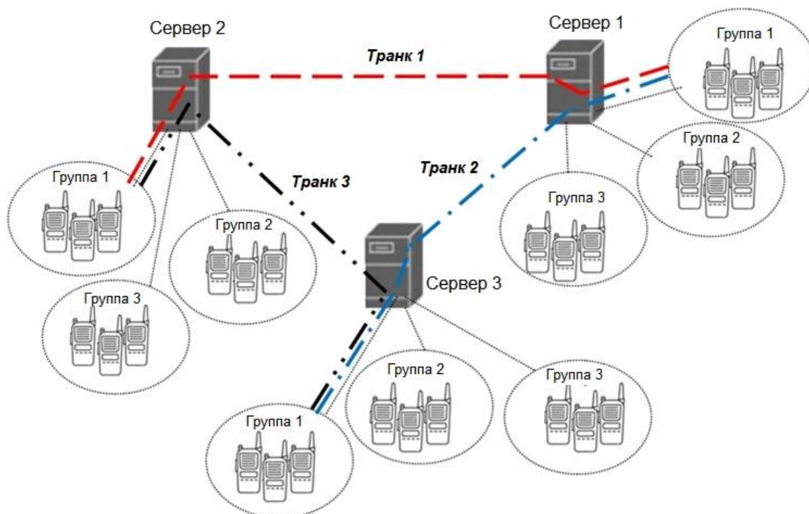
Рис. 3: Мультисерверная система с «Глобальной» абонентской группой
