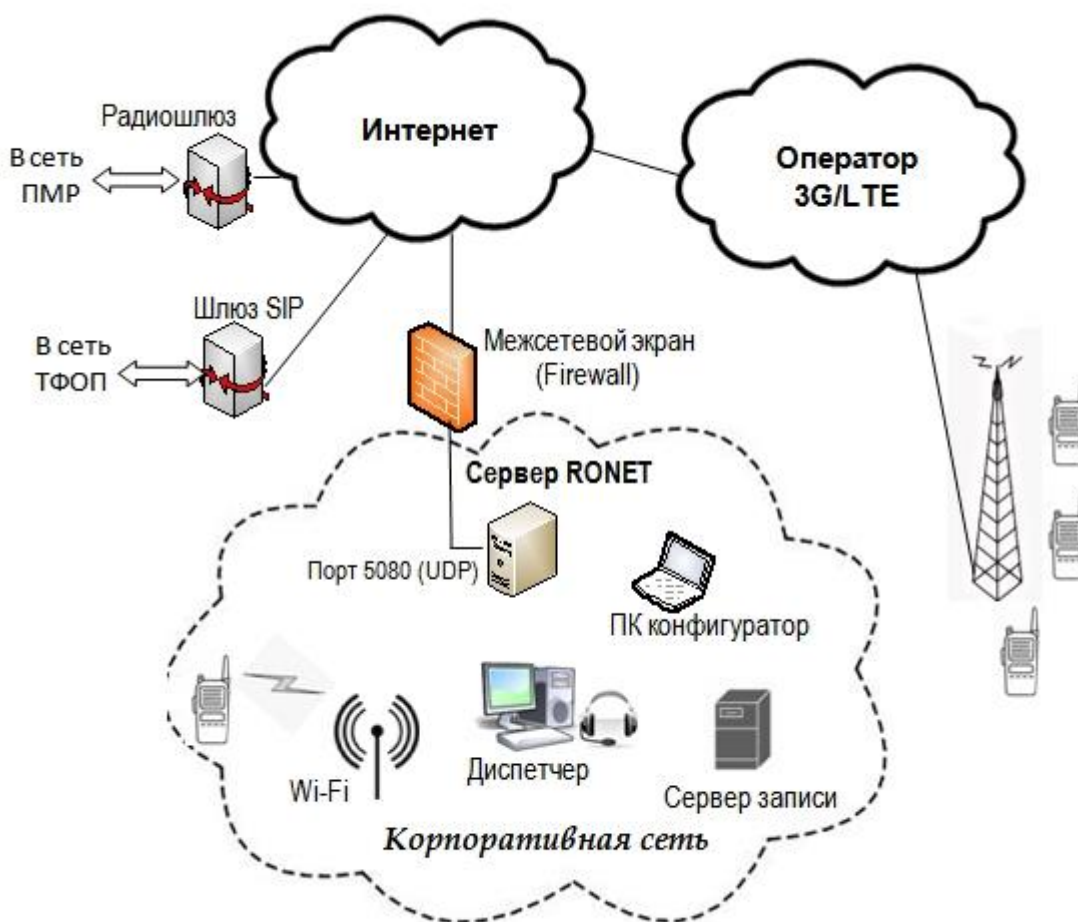
Рис. 1 Общая схема системы
